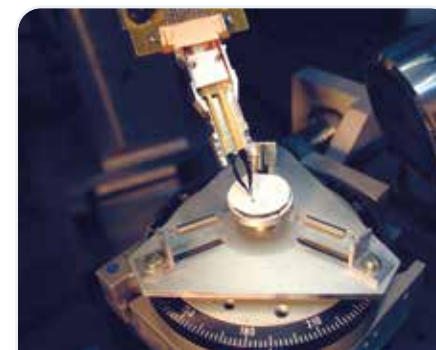
↑ Chronogrip, micro-pince pour manipuler des objets miniatures ©Percipio Robotics
